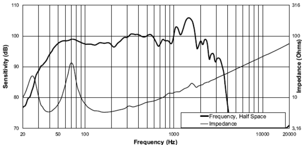
Ilustracja 2: Zakres częstotliwości
