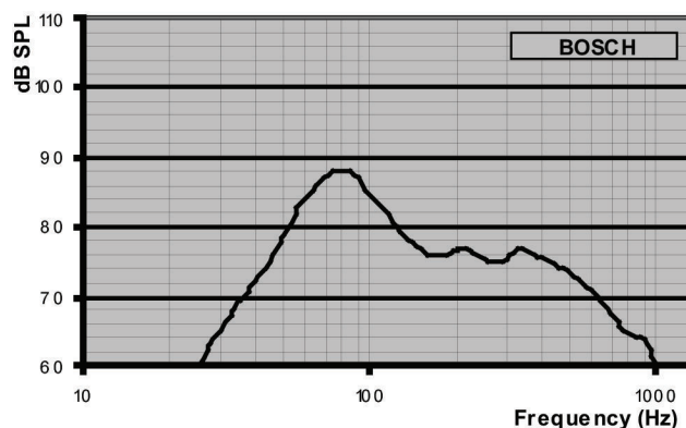
LB1-SW60 Pasmo przenoszenia
