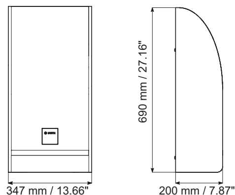
LB1-SW60 Wymiary
