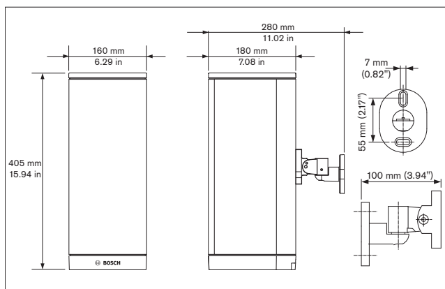
Wymiary
