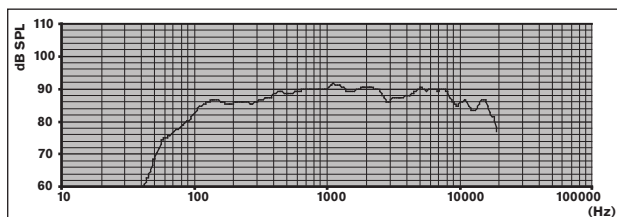
Pasmo przenoszenia
