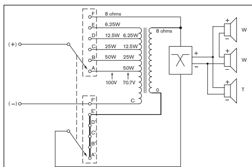
Schemat połączeń
