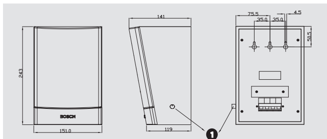
Wymiary głośników LB1-UW06-x z regulacją głośności (1)
