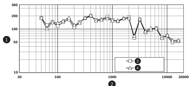
Pasma przenoszenia
