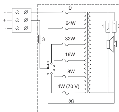
Schemat połączeń (1: filtr dolnoprzepustowy, 2: filtr górnoprzepustowy, 3: bezpiecznik termiczny)
