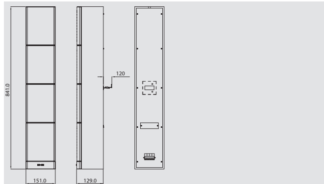
Wymiary
