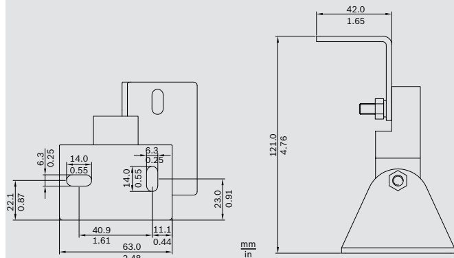
Wymiary wspornika
