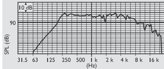
Pasma przenoszenia
