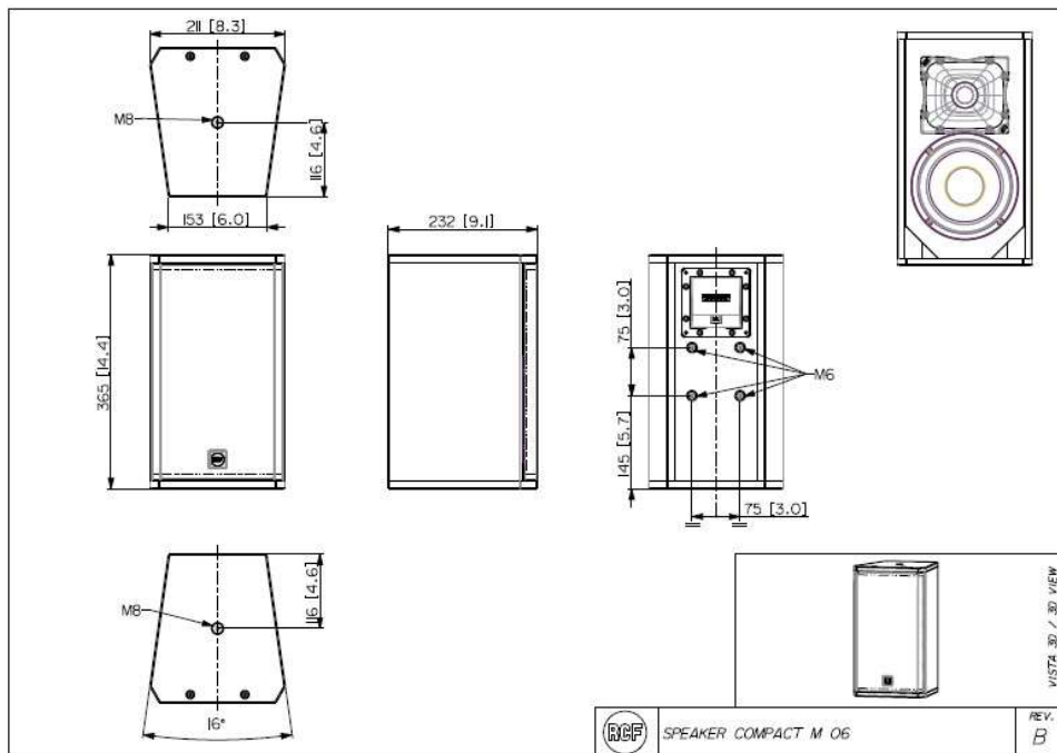
Rysunek techniczny 2D
