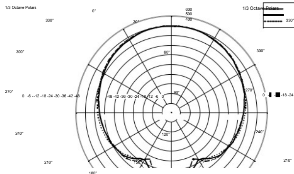
1/3 Octave Polars
