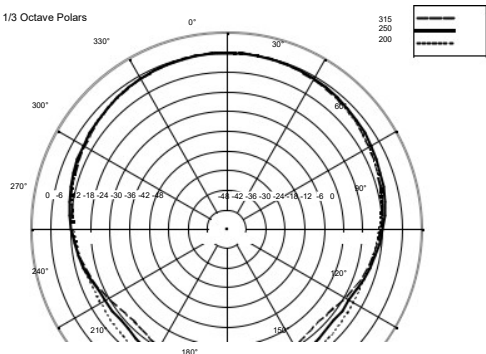
1/3 Octave Polars
